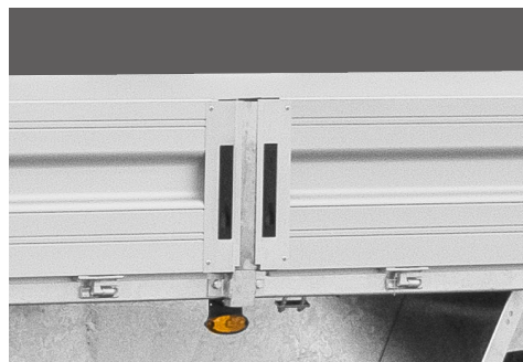
Montierte Mittelrungen an den seitlich geteilten Bordwänden (ab 6100 mm Innenlänge)
