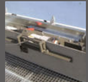
Seilwinde auf der Ladefläche
