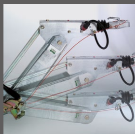
Höhenverstellbare Zugdeichsel (Kugelpfropf und DIN Zugöse nicht inklusive)
