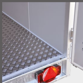
Bodenplatte mit Alu-Riffelblech belegt
