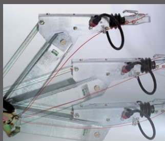
Höhenverstellbare Zugdeichsel (Kugelpf-Kupplung und DIN-Zugöse nicht inklusive)
