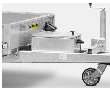
Deichselbox zum Schutz der Batterie und der Absenkhidraulik
