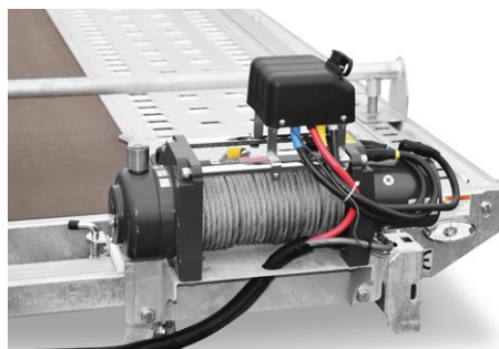
Elektrische Seilwinde
